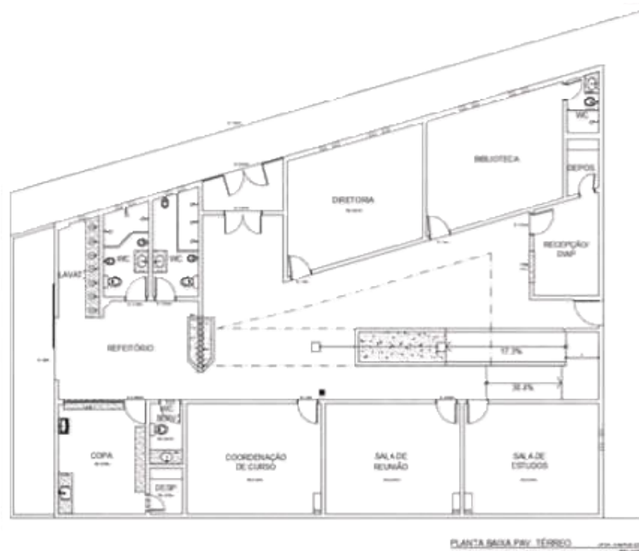
Figura 17 – Campus Icó - Plantas Baixa do Pavimento Térreo e Primeiro Andar Fonte: Diretoria de Infraestrutura - Universidade Federal do Cariri – Ano 2017
