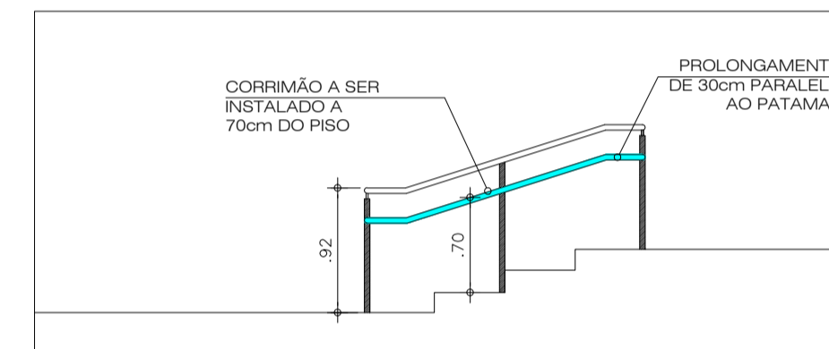
9 CORRIMÃO INTERMEDIÁRIO ESCADA ENTRE BLOCO B e D ESCALA 1/50
