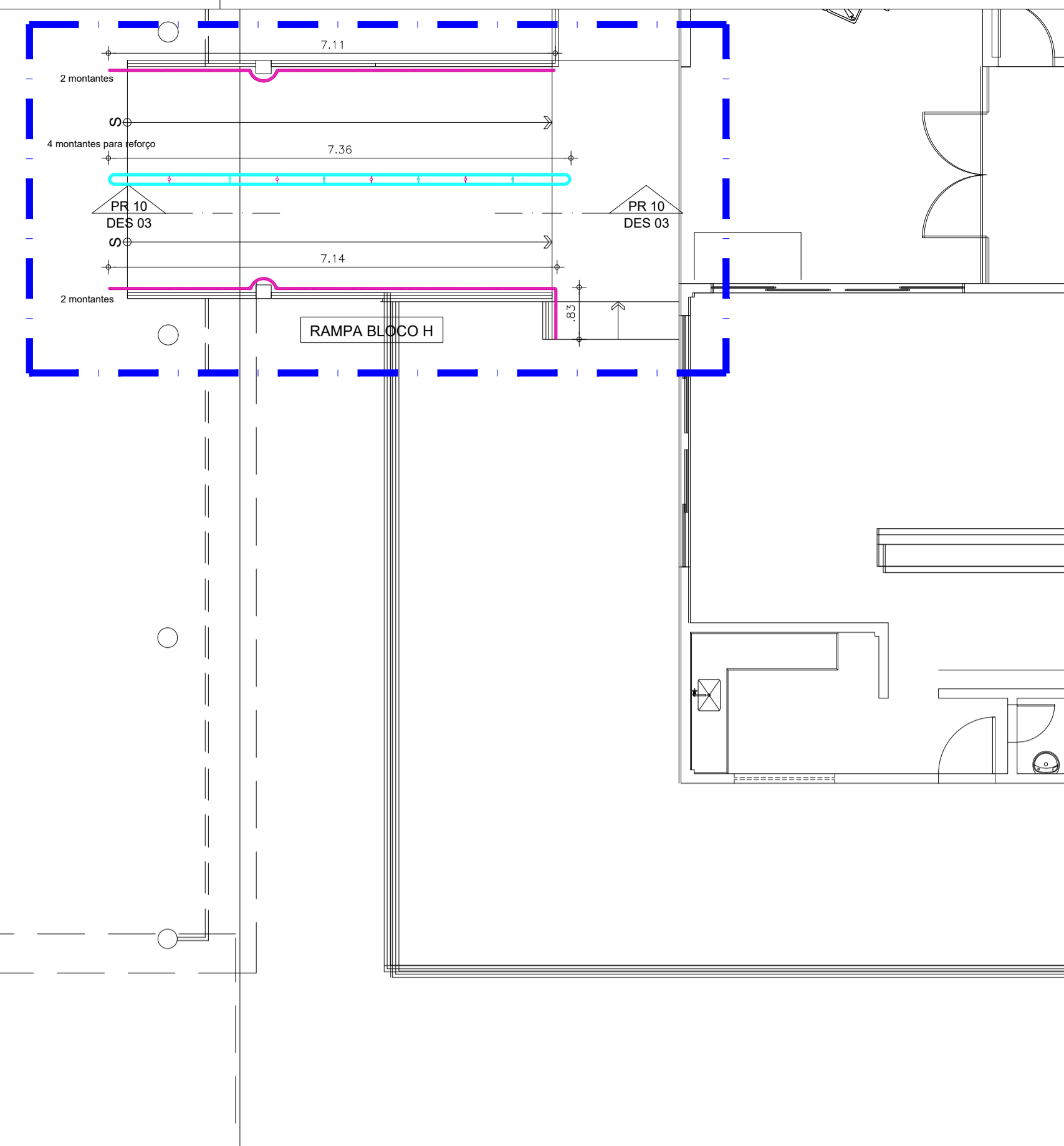
1 PLANTA DE CORRIMÃOS - G E H ESCALA 1/75
