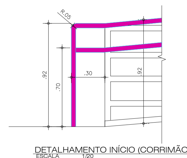
DETALHAMENTO INÍCIO (CORRIMÃO) ESCALA 1/20
