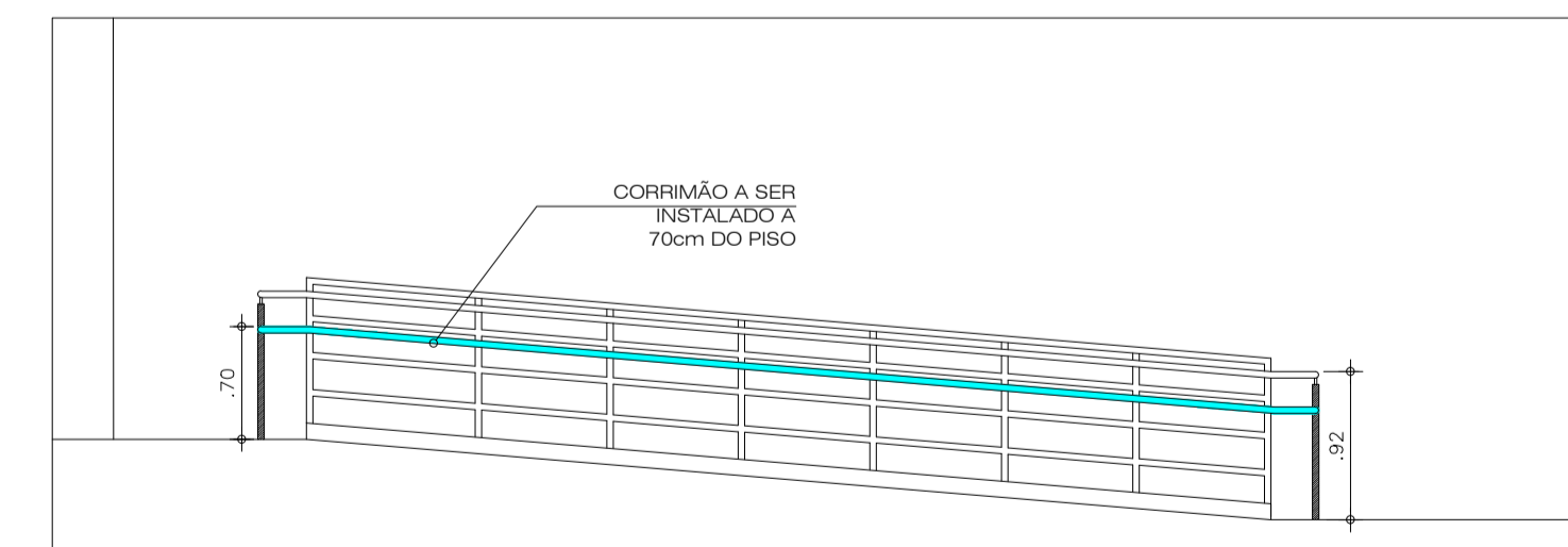
13 CORRIMÃO INTERMEDIÁRIO RAMPA BLOCO E ESCALA 1/50
