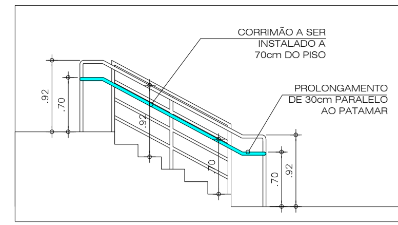
2 CORRIMÃO EXTREMIDADES - ESCADA GUARITA ESCALA 1/50
