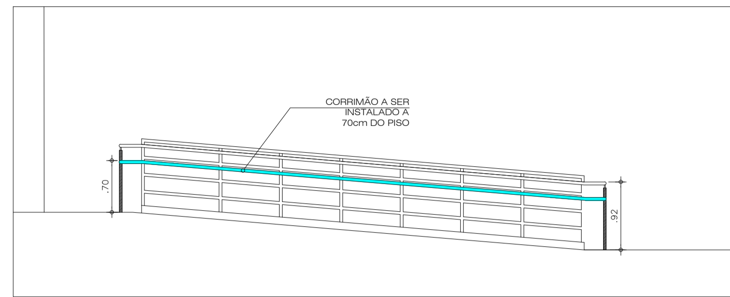
1 CORTE - RAMPA BLOCO G ESCALA 1/50
