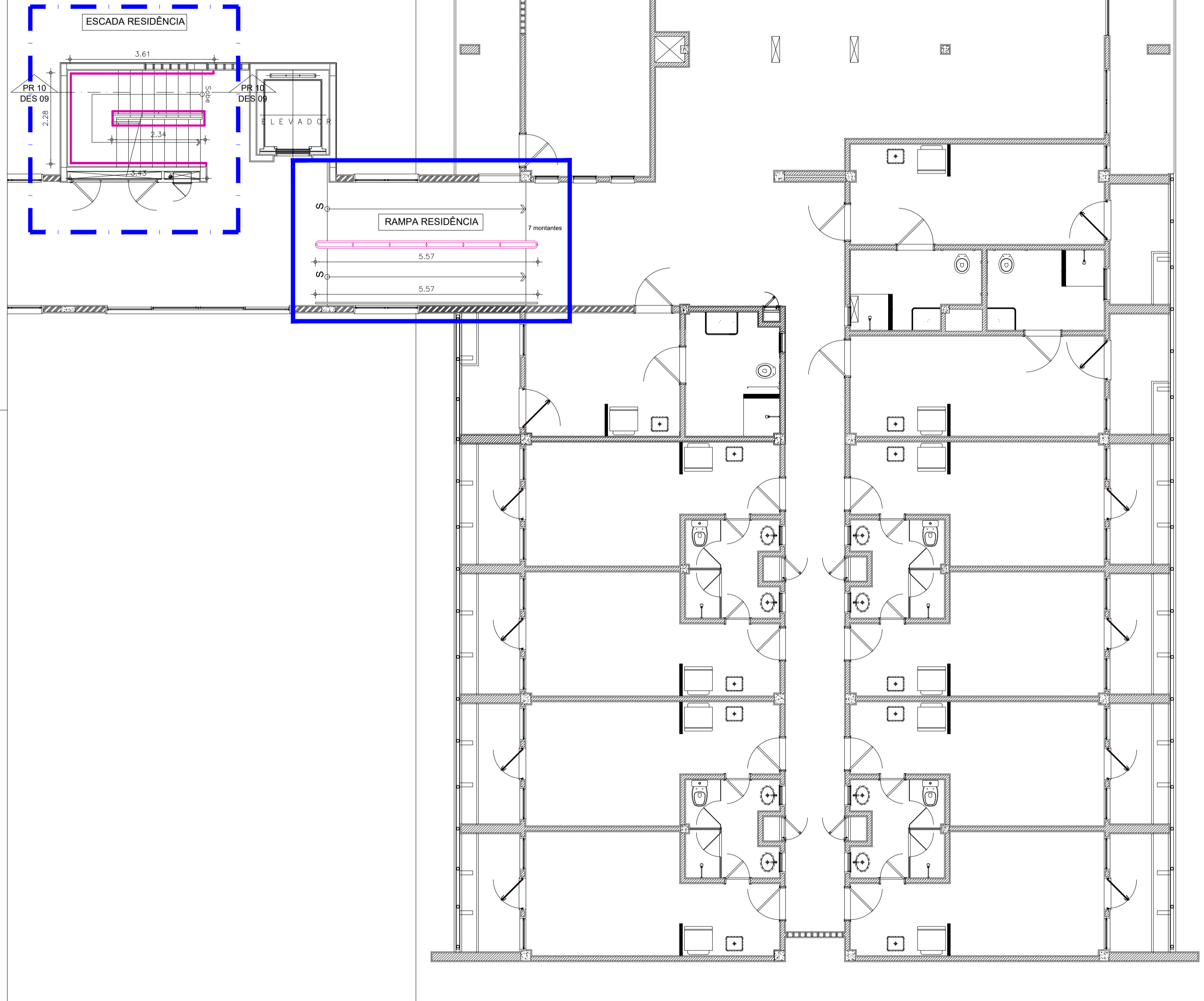
1 PLANTA DE CORRIMÃOS - RESIDÊNCIA TÉRREO ESCALA 1/75
