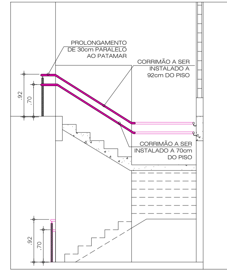
2 CORTE - ESCADA BLOCO G ESCALA 1/50
