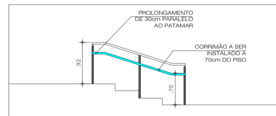
8 CORRIMÃO ESCADA ENTRE BLOCO B e D ESCALA 1/50
