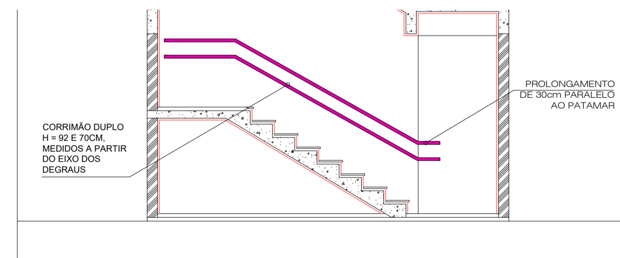
9 CORRIMÃO ESCADA - RESIDENCIA ESCALA 1/50
