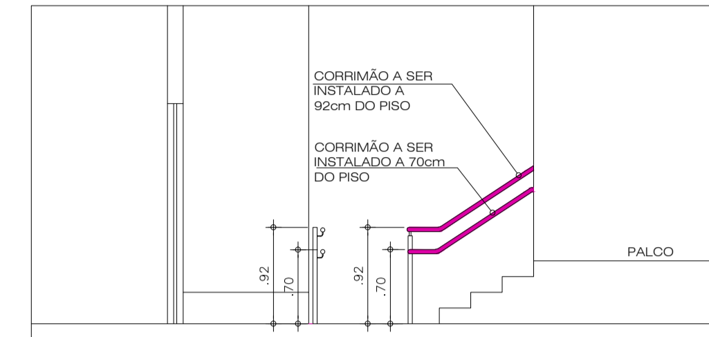
5 CORRIMÃO ESC. INTERNA PALCO - BLOCO H ESCALA 1/50
