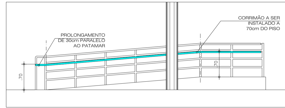
3 CORRIMÃO EXTREMIDADES - RAMPA GUARITA ESCALA 1/50
