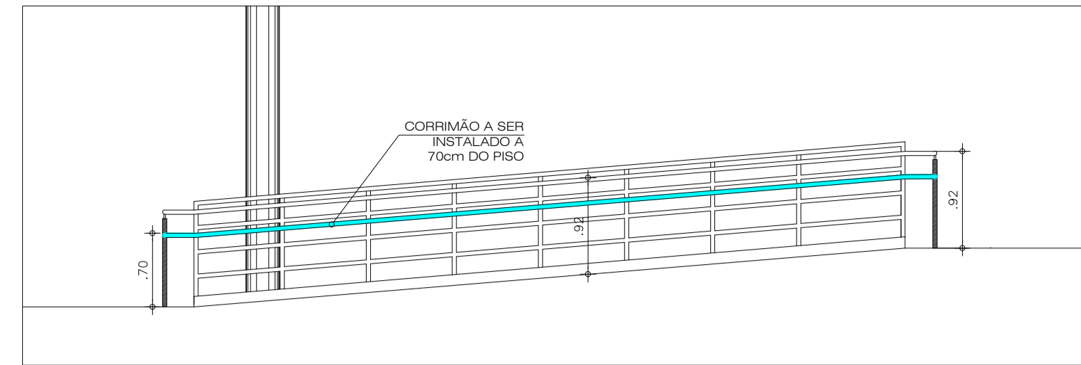
3 CORRIMÃO RAMPA BLOCO H ESCALA 1/50
