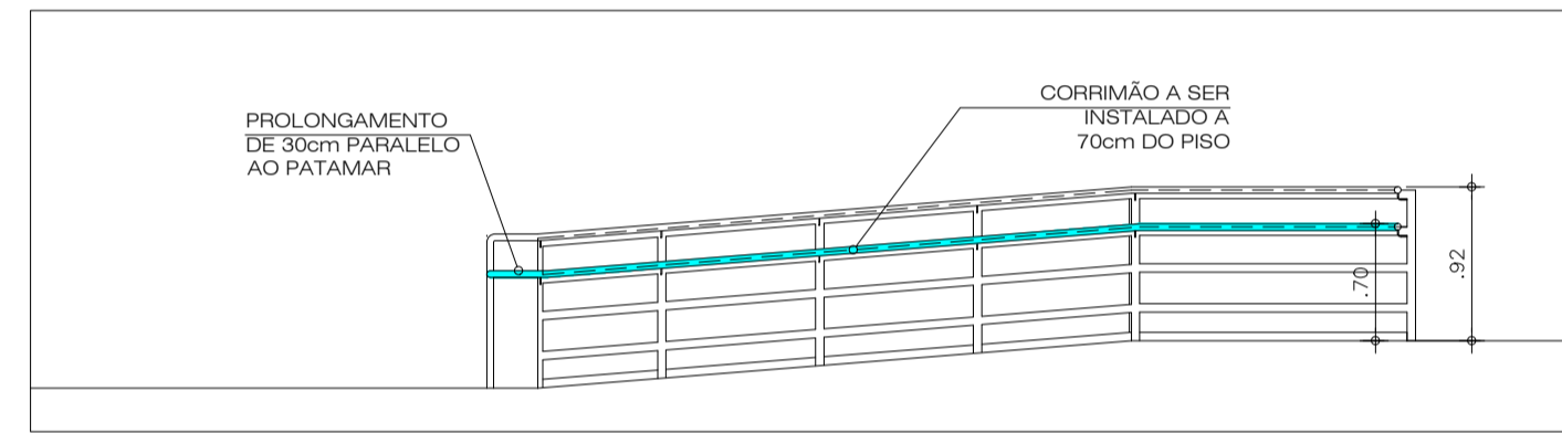
6 CORRIMÃO RAMPA BLOCO B - PRIMEIRO SEGMENTO ESCALA 1/50
