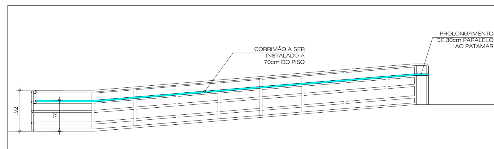
12 CORRIMÃO SEGUNDO SEGMENTO DA RAMPA BLOCO D ESCALA 1/50
