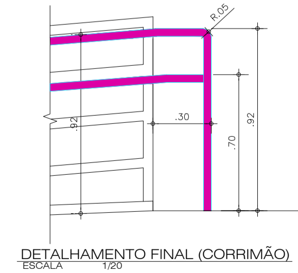
DETALHAMENTO FINAL (CORRIMÃO) ESCALA 1/20
