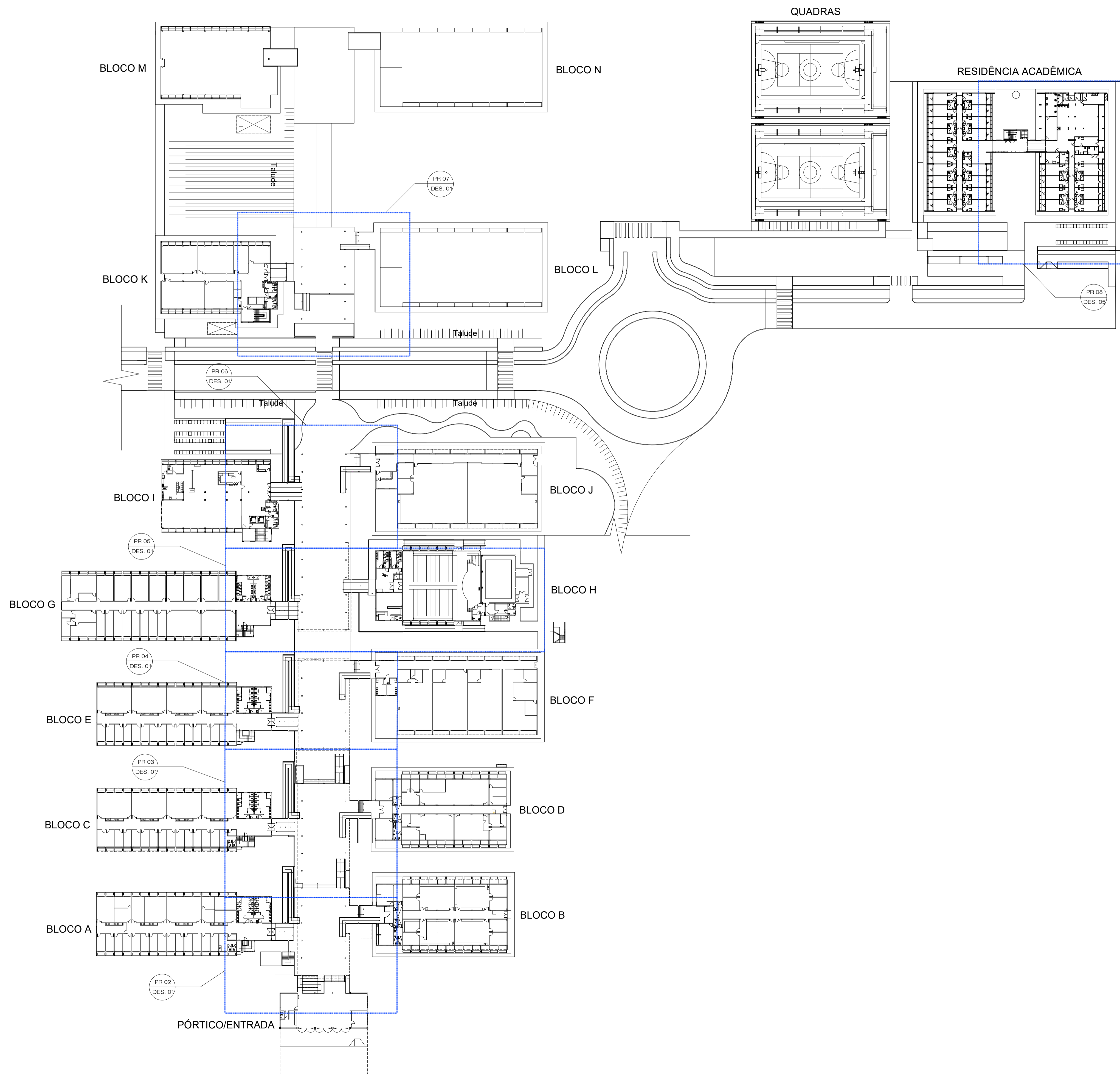
1 PLANTA GERAL SEM ESCALA
