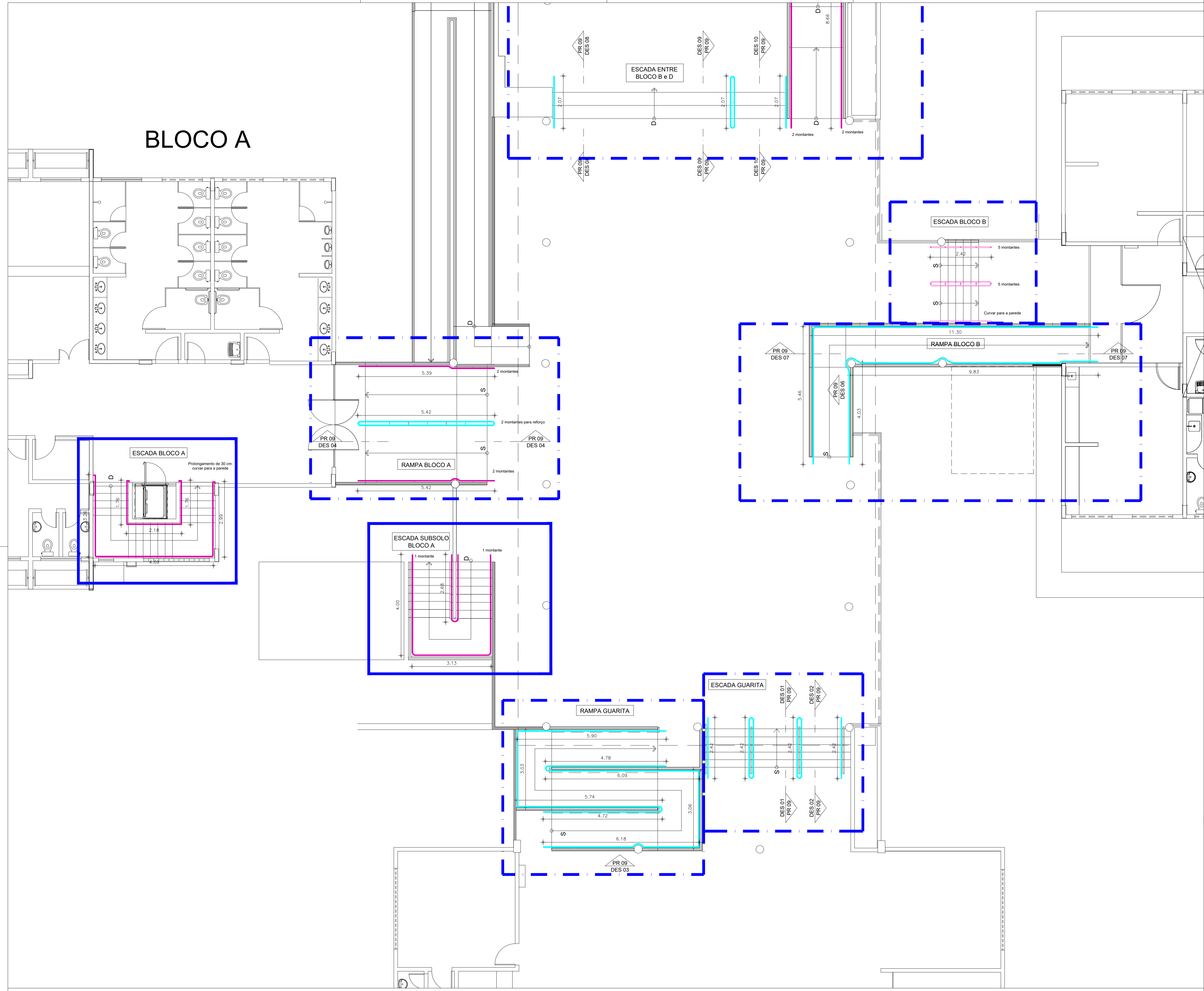
1 PLANTA DE CORRIMÃOS - GUARITA, BLOCO A E B ESCALA 1/75
