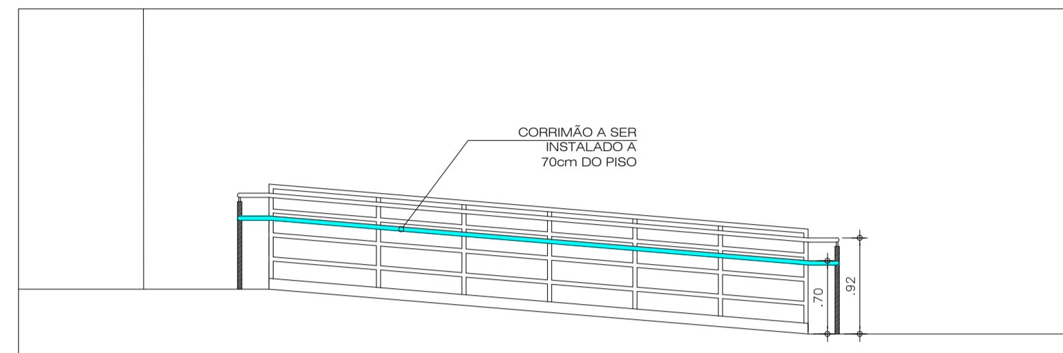
5 CORRIMÃO INTERMEDIÁRIO RAMPA BLOCO C ESCALA 1/50
