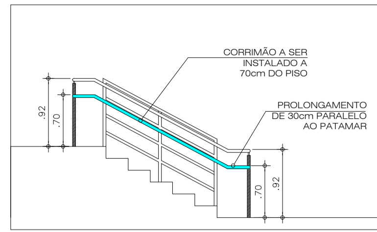
1 CORRIMÃO CENTRAL - ESCADA GUARITA ESCALA 1/50
