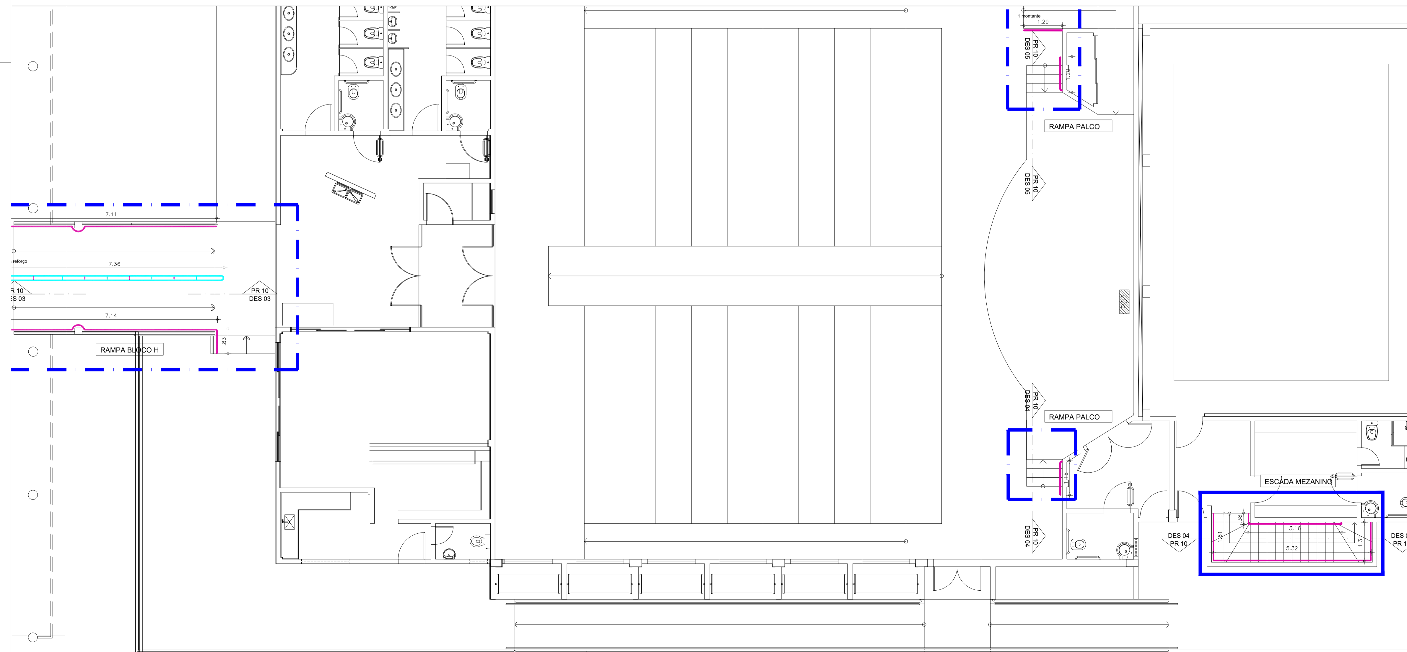
2 PLANTA DE CORRIMÃOS - H (interno) ESCALA 1/75
