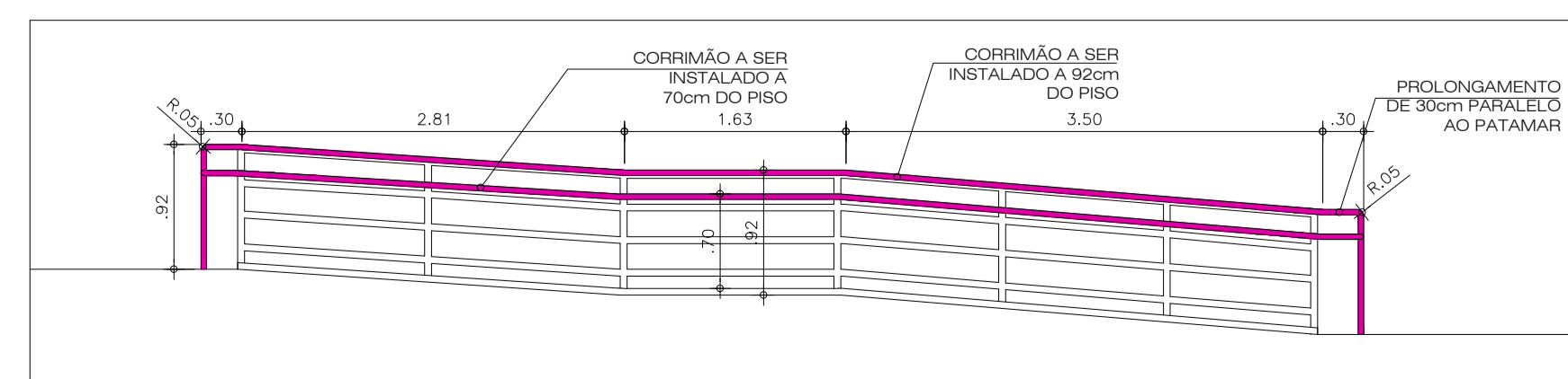
14 CORRIMÃO RAMPA ENTRE BLOCO D e F ESCALA 1/50
