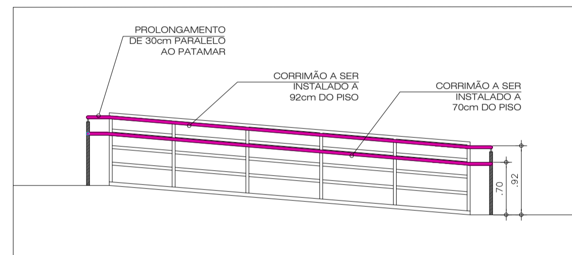
6 CORRIMÃO RAMPA BLOCO I e K ESCALA 1/50
