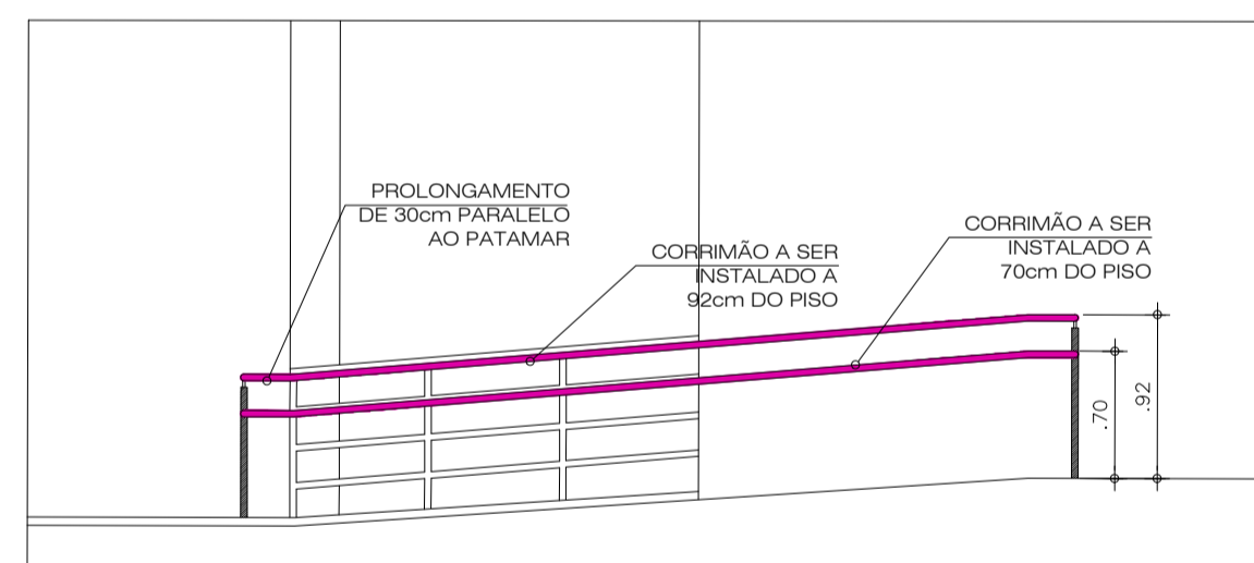
7 CORRIMÃO RAMPA BLOCO K ESCALA 1/50
