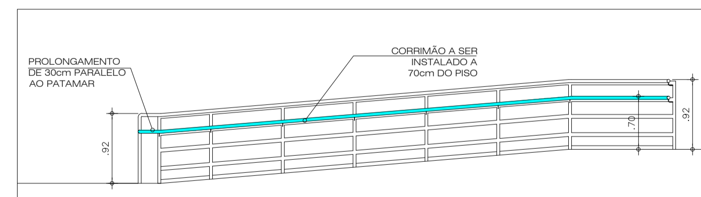
11 CORRIMÃO PRIMEIRO SEGMENTO DA RAMPA BLOCO D ESCALA 1/50
