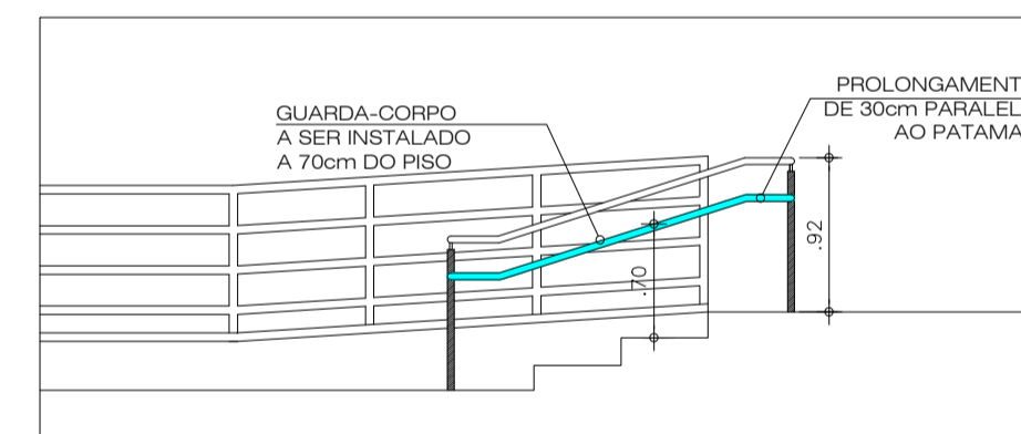
10 CORRIMÃO ESCADA ENTRE BLOCO B e D ESCALA 1/50
