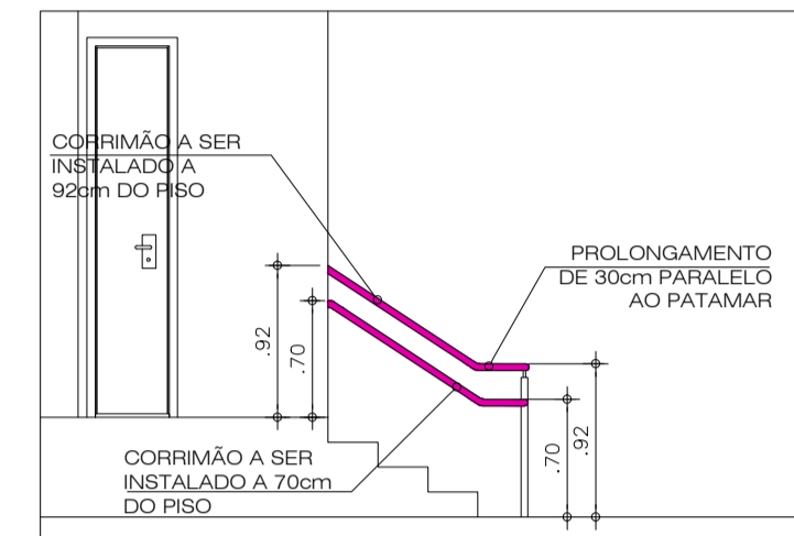
4 CORRIMÃO ESC. INTERNA PALCO - BLOCO H ESCALA 1/50
