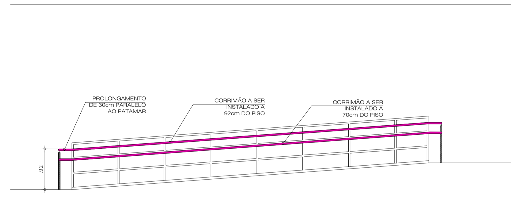
8 CORRIMÃO RAMPA BLOCO L ESCALA 1/50
