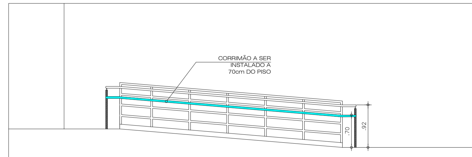
4 CORRIMÃO INTERMEDIÁRIO RAMPA BLOCO A ESCALA 1/50
