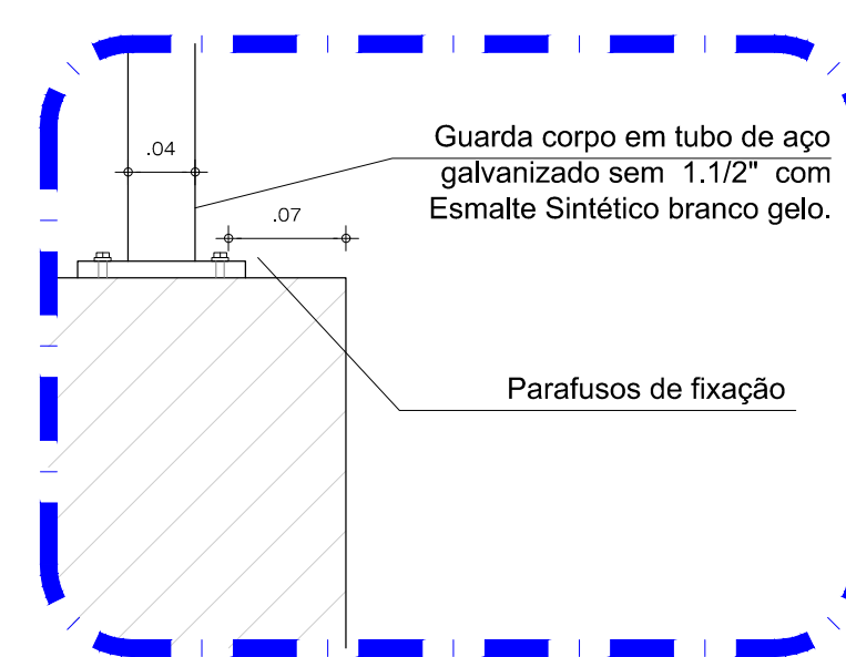
03 DET. FIXAÇÃO DO GUARDA-CORPO NA PASSARELA
