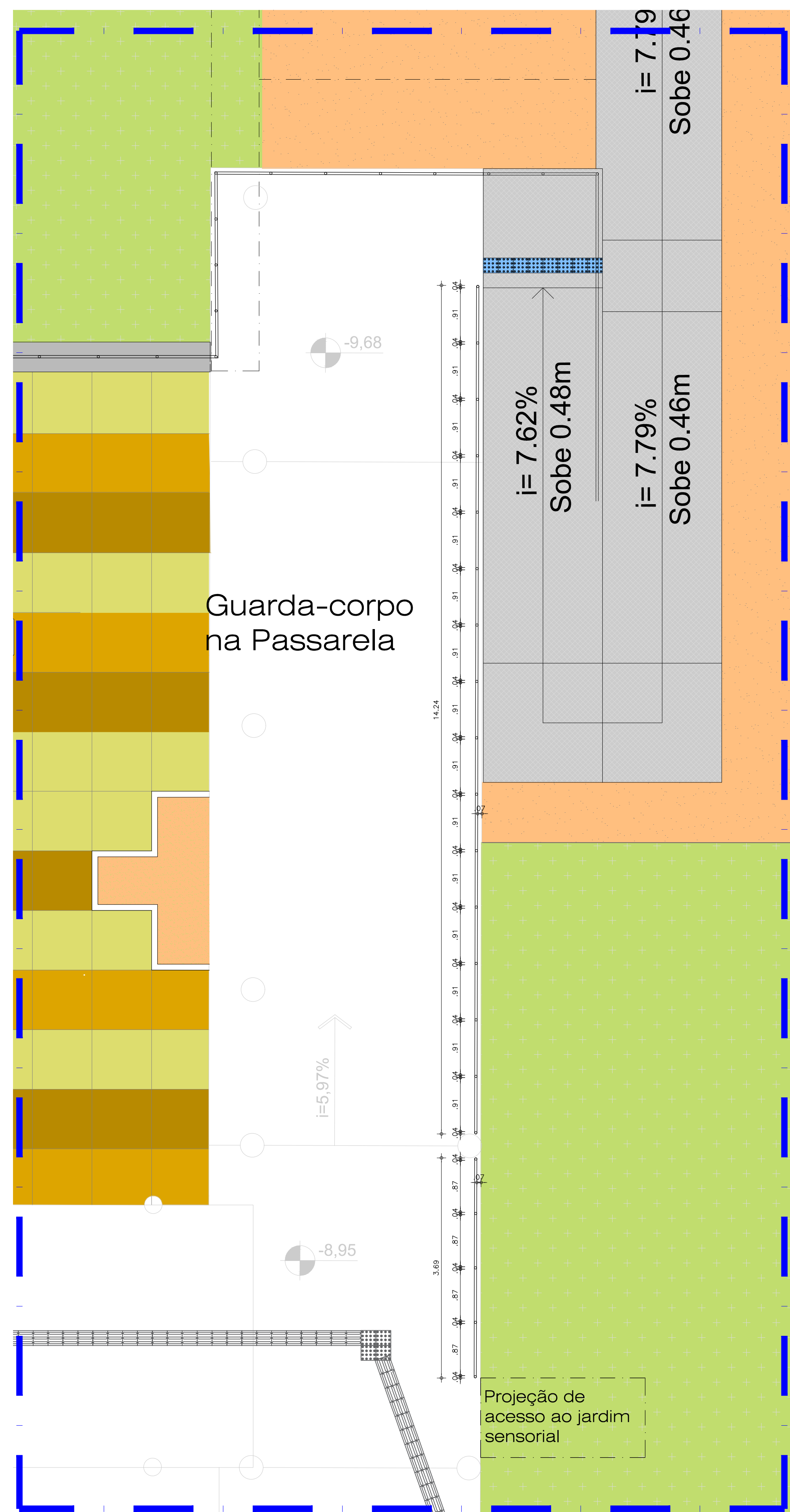
01 PLANTA BAIXA MONTANTES E GUARDA-CORPO
