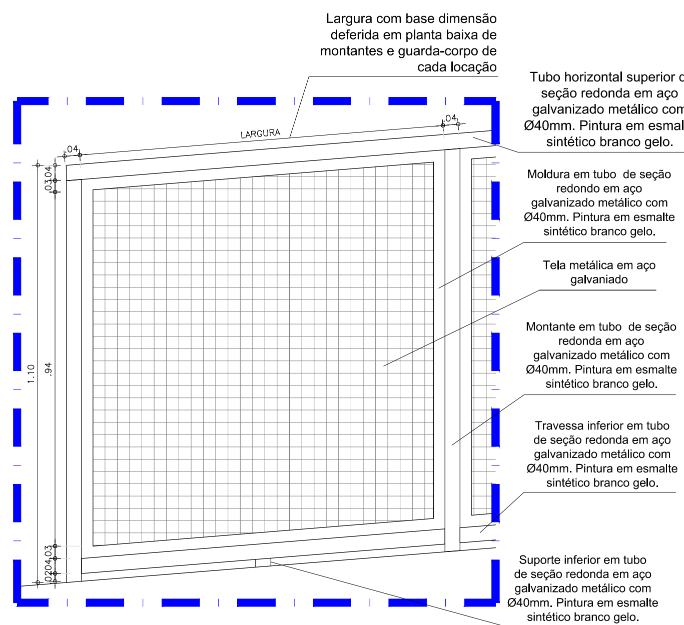
02 DETALHE GUARDA-CORPO
