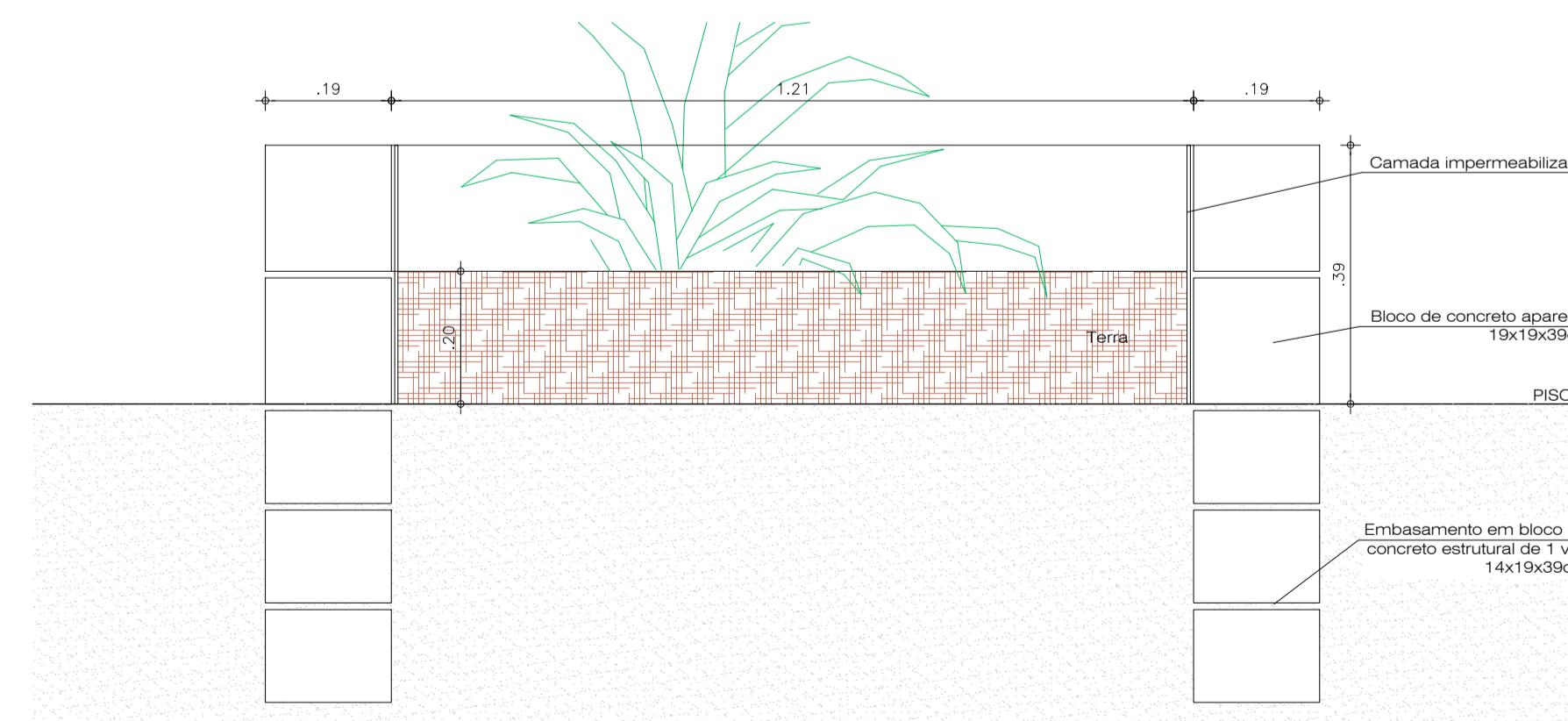
3 DETALHE - JARDINEIRAS ESPAÇO DIDÁTICO ESCALA 1/10
