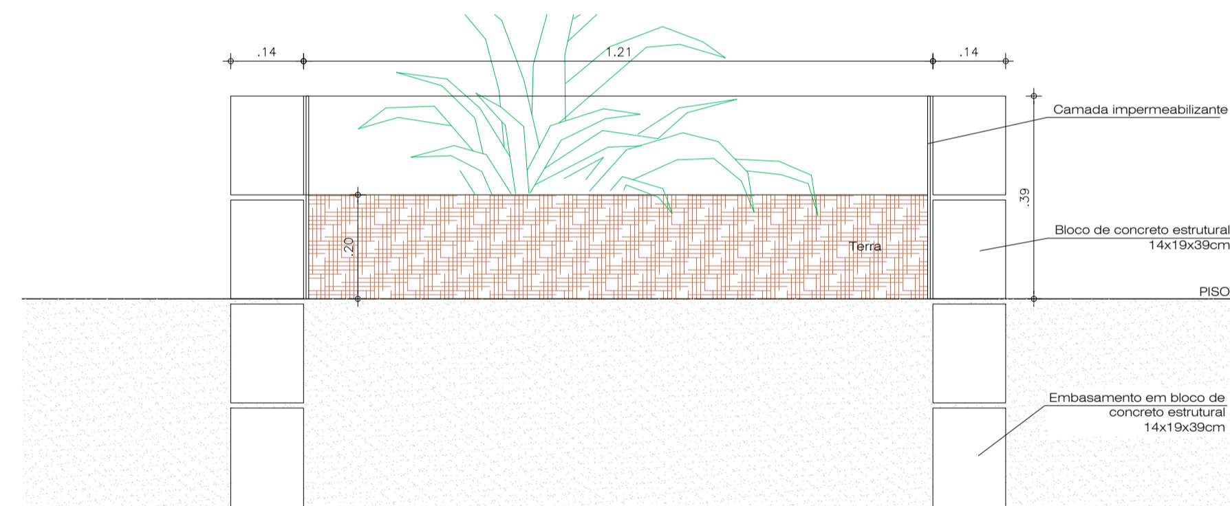
2 DETALHE - JARDINEIRAS HORTO ESCALA 1/10
