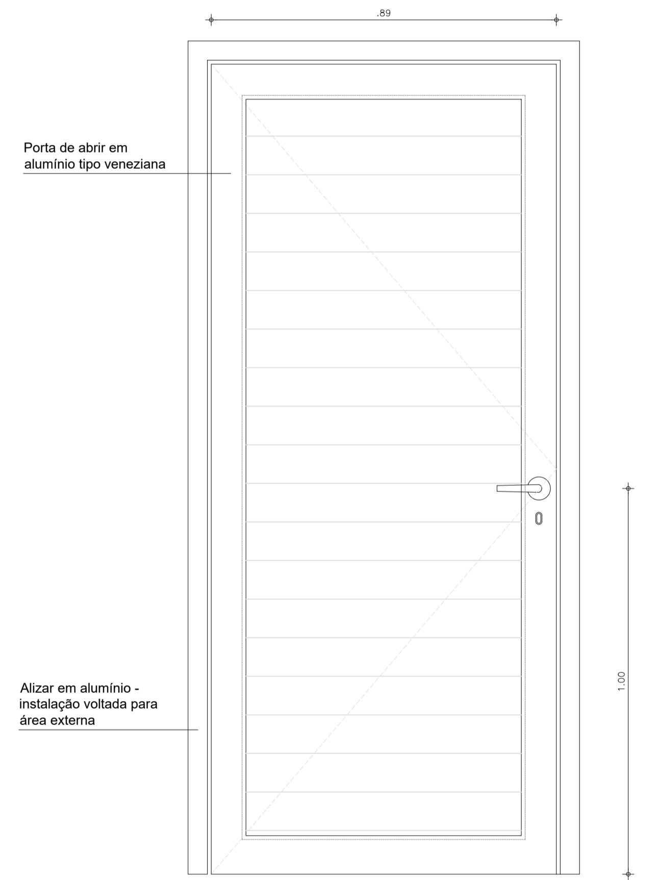
4 DETALHE P3 - PORTA DEPÓSITO ESCALA 1/10
