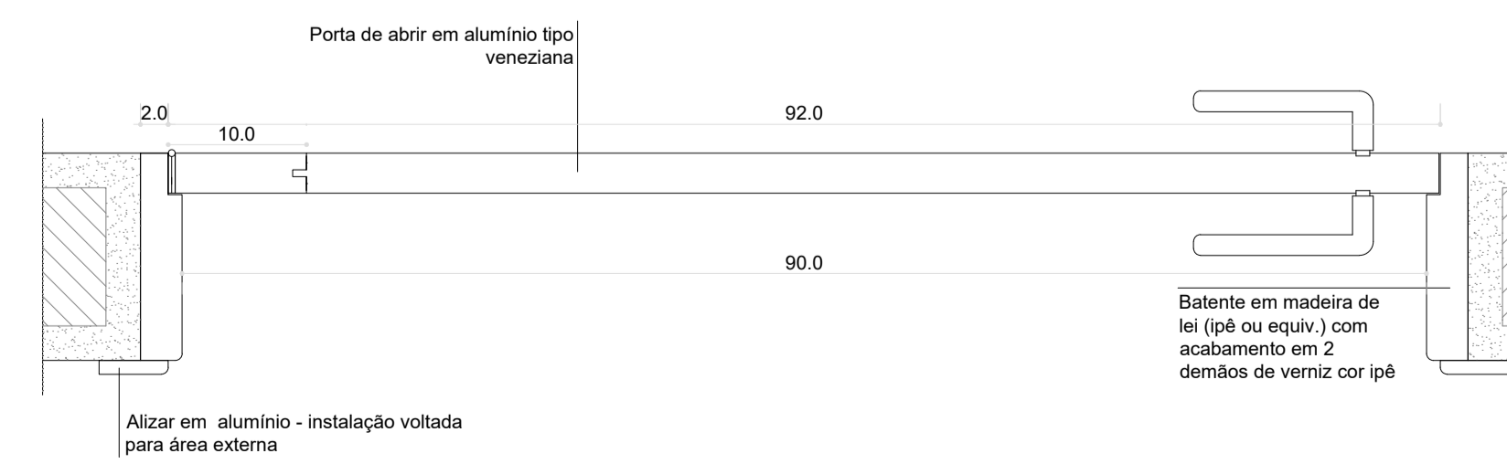
5 DETALHE P3 - PLANTA BAIXA PORTA DEPÓSITO ESCALA 1/5
