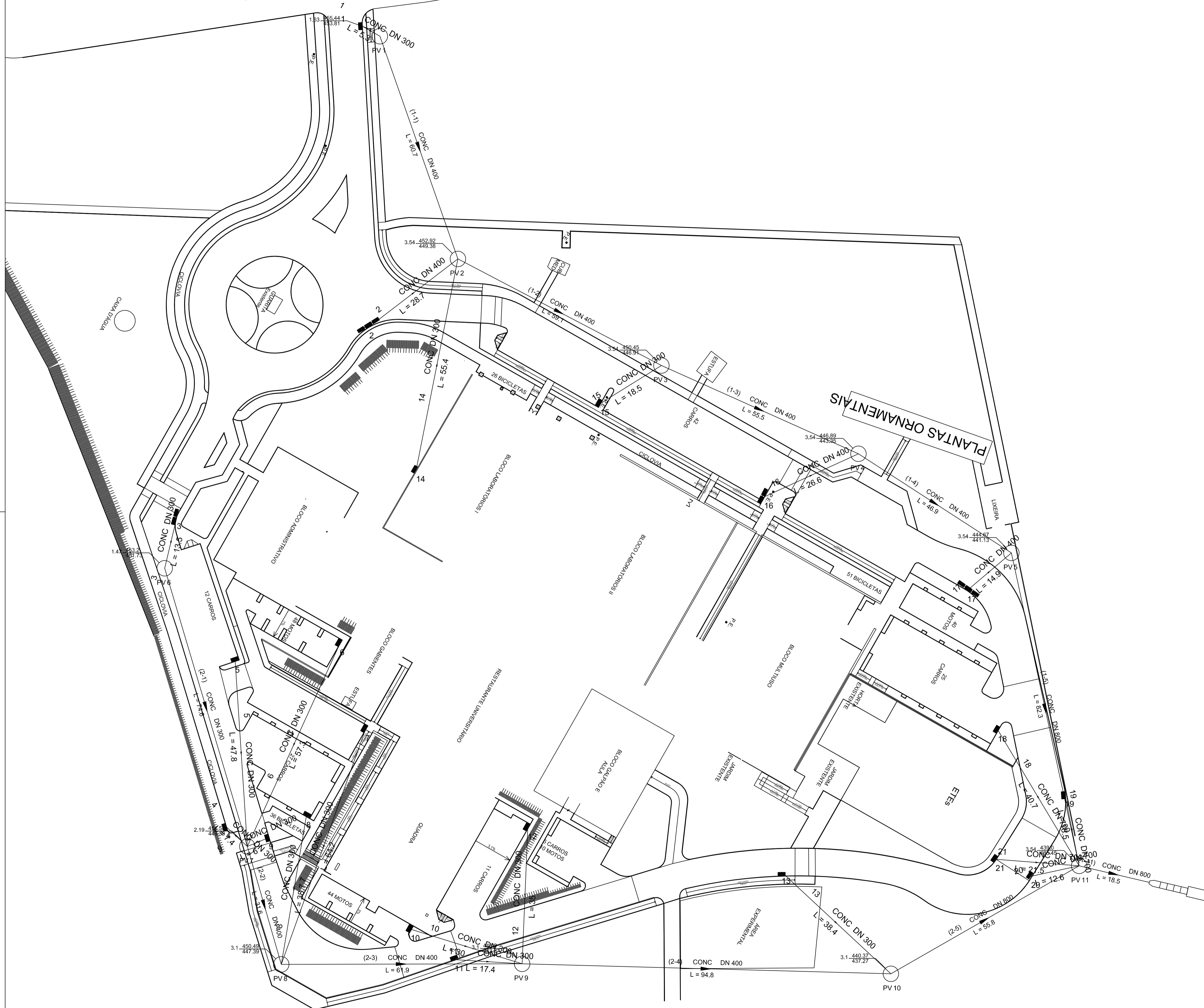
1 PROJETO DE MICRODRENAGEM ESCALA 1/500
