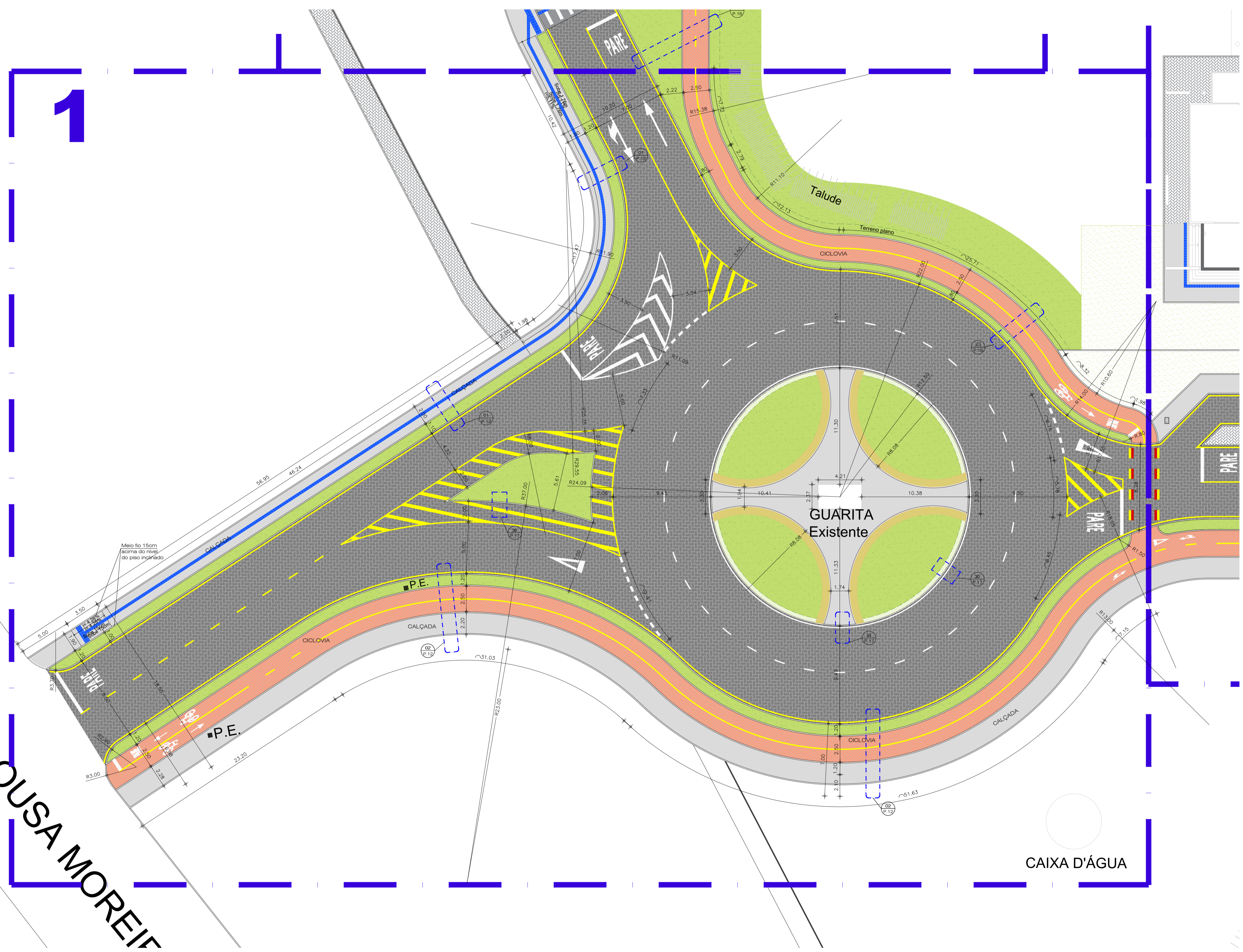
1 AMPLIAÇÃO QUADRANTE 1 ESCALA 1/200
